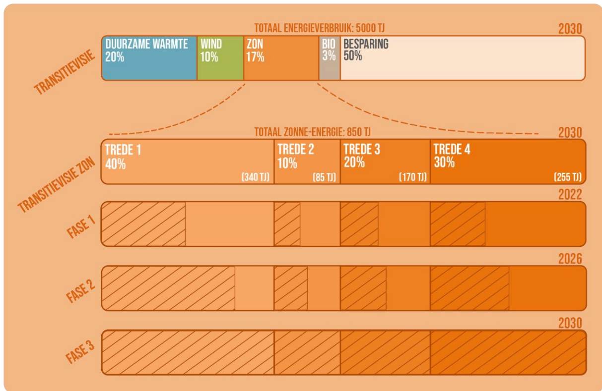
Figuur 3 - Fasering van de transitieopgave zonne-energie voor een fictieve gemeente
